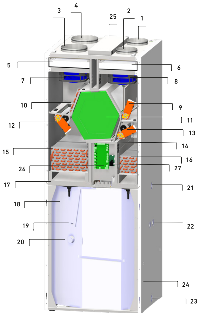
PKOM 4 A/AK CLASSIC (RECHTE AUSFÜHRUNG)
