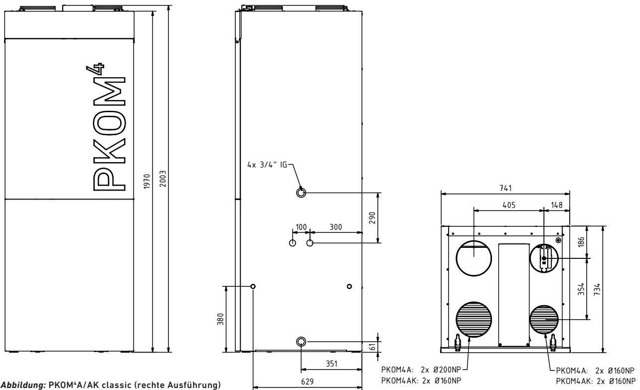
Abbildung: PKOM 4 A/AK classic (rechte Ausführung)
