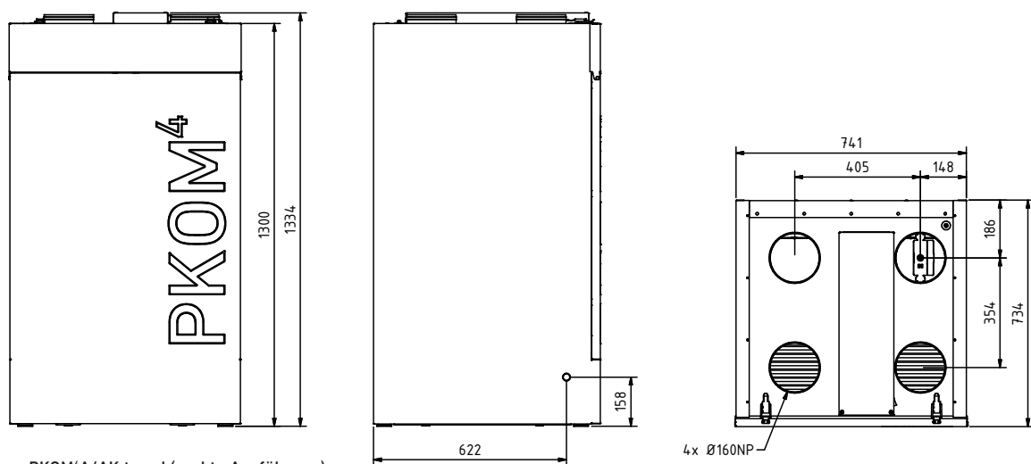
Abbildung: PKOM 4 A/AK trend (rechte Ausführung)
