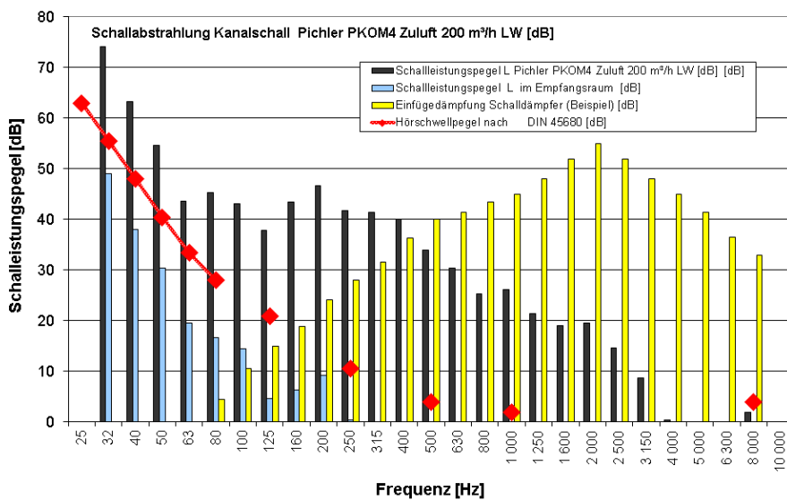
Abbildung 2: Schallabstrahlung Zuluftkanal
