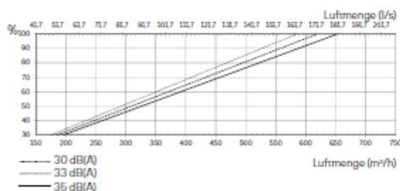
Kapazität mit ePM 10 55% + ePM 10 50% Filter 1
