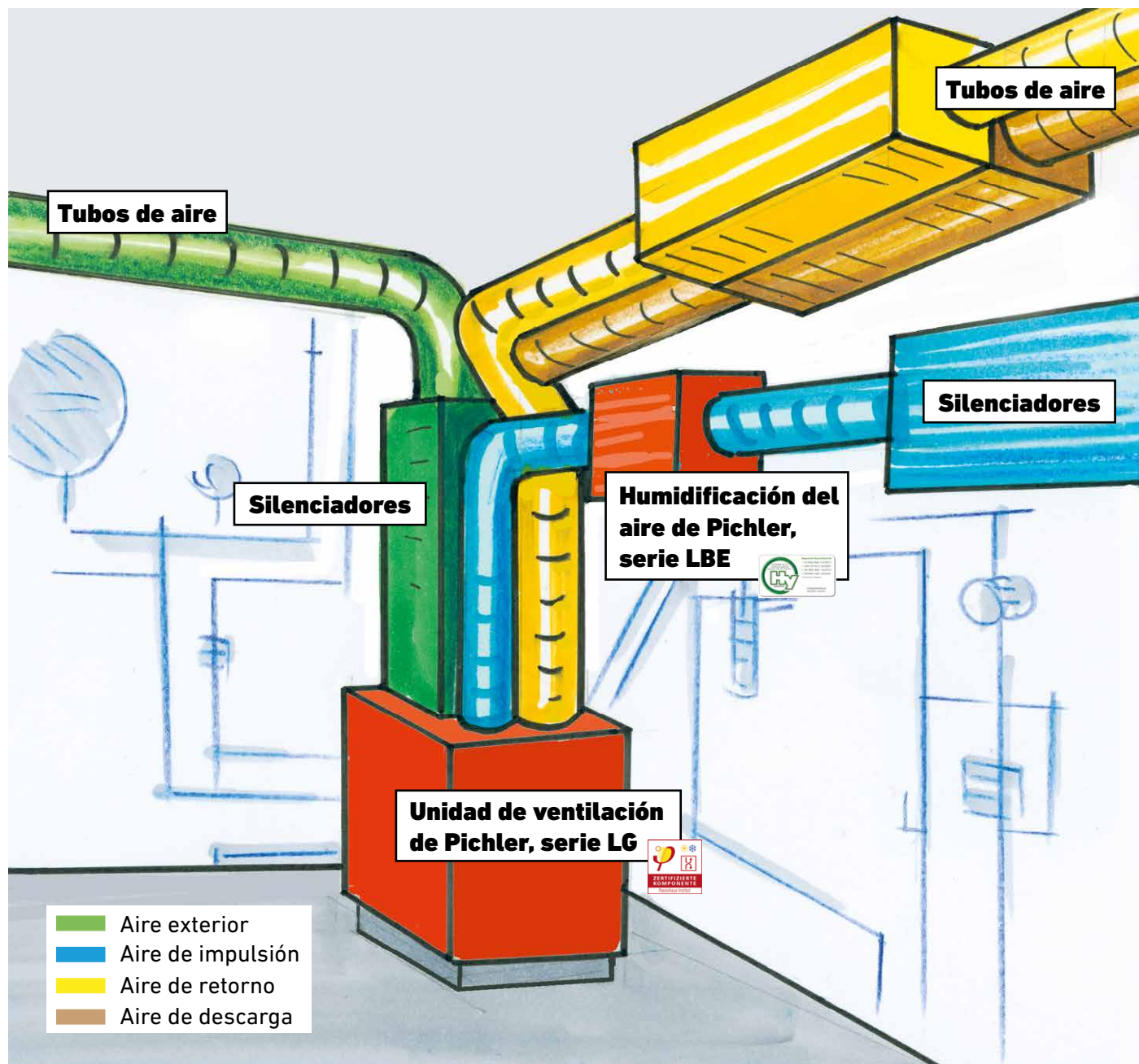
Figura del esquema de la instalación: Representación de su sistema de ventilación en la sala de calefacción o técnica, con el panel de control colocado en el salón de casa: para un clima saludable con una humedad óptima durante todo el año.
