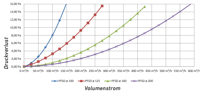
Druckverlust
