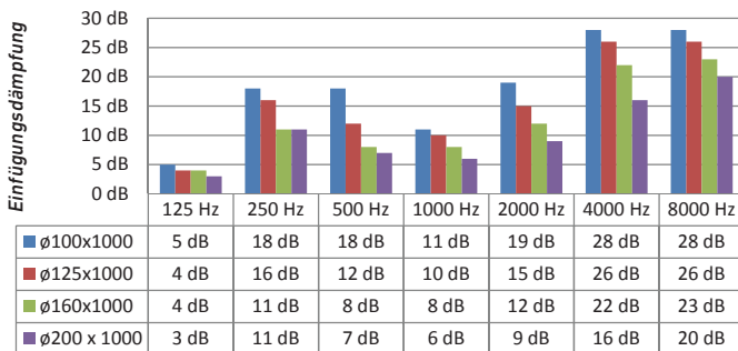
Einfügungsdämpfung PFSD Ø 100 - 200 l = 1000 mm
