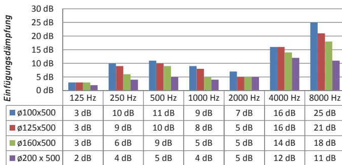
Einfügungsdämpfung PFSD Ø 100 - 200 l = 500 mm
